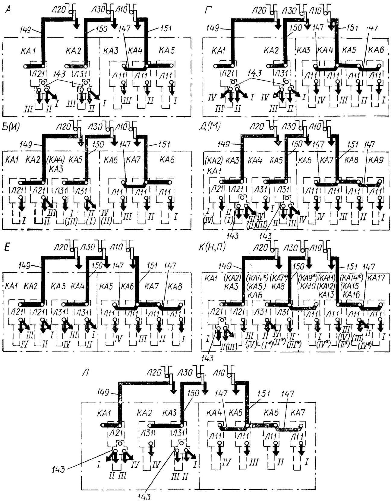
Схема электрическая соединений электромагнитов реле РЗО-401 для защитных панелей ПЗКБ-160У2, ПЗКБ-250У2.
